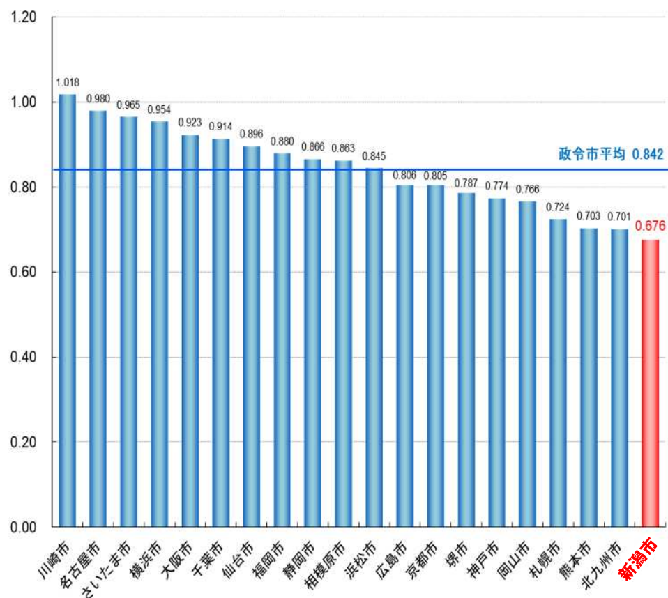
財政力指数
