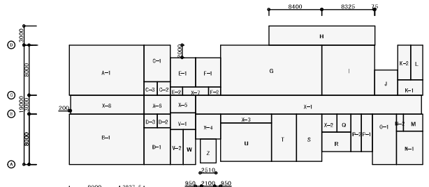
1階求積図
