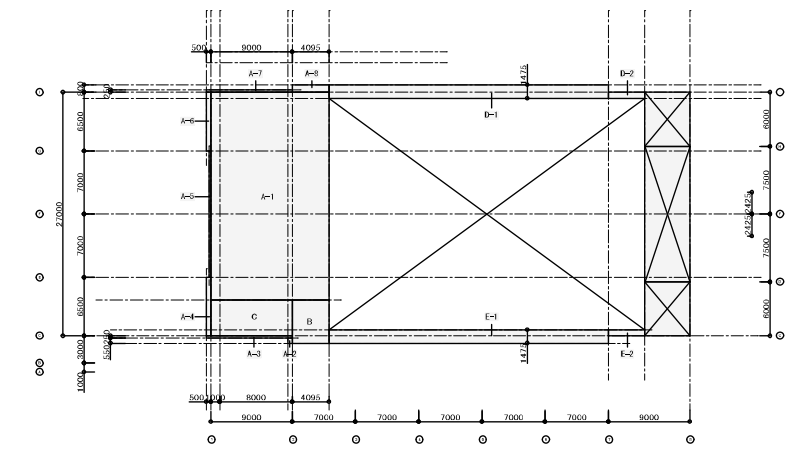
体育館2階求積図
