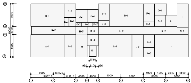
2階求積図
