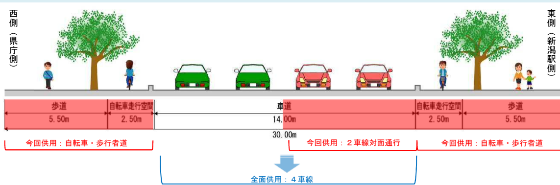
〔標準横断面図 (4車線完成時)〕
