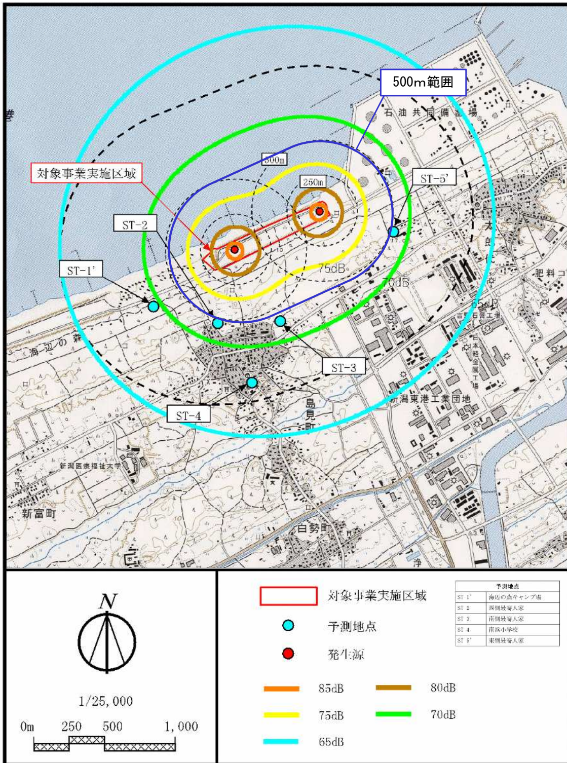
図 13 施設の稼働に係る低周波音の等騒音線図
