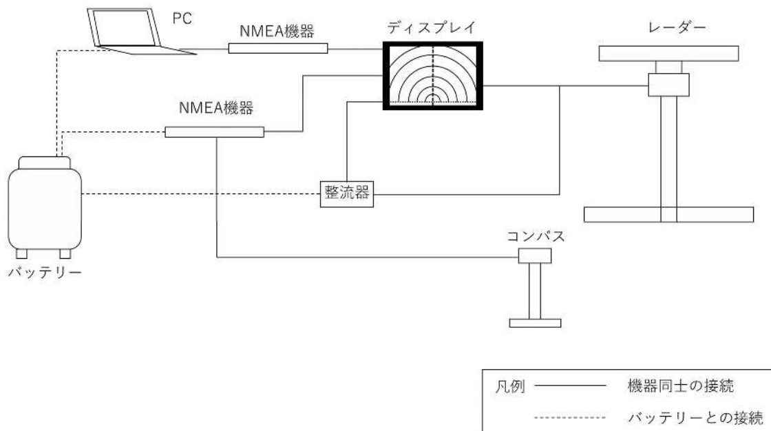
図 8 機器構成図
