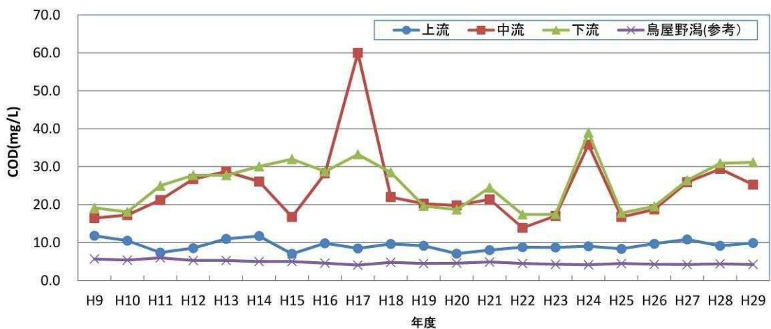
図16 CODの年平均値
