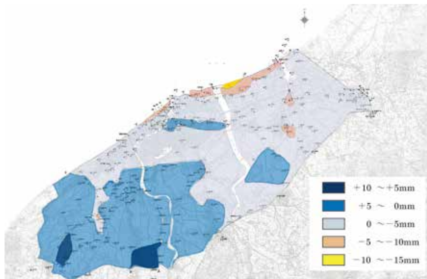
図表5-6 新潟・新発田地域地盤変動図 (H30.9.1-R1.9.1)
