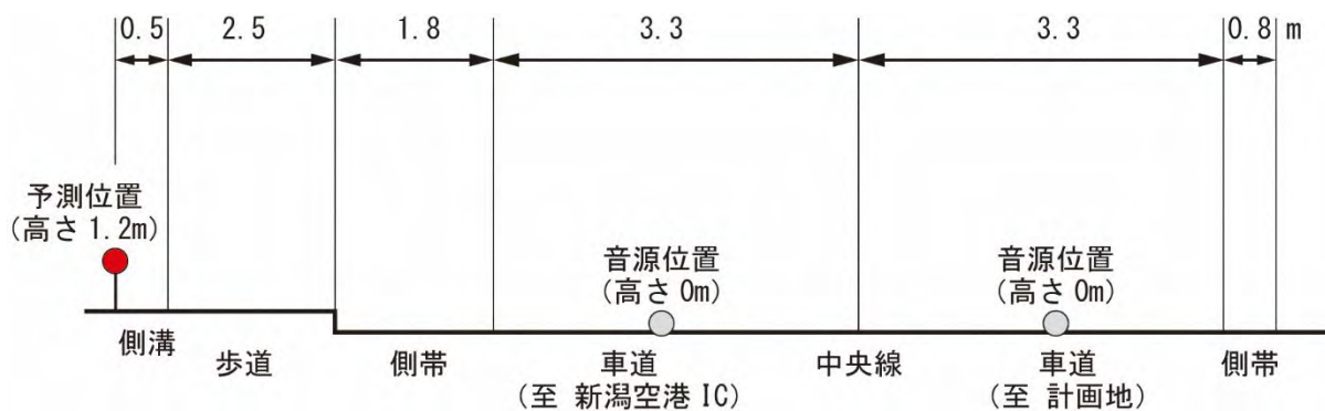
図 7.2.12(3) 道路断面図 (No.3 : 嘉瀬蔵岡線沿道 (東側))
