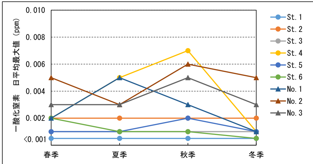
図 7.1.4 一酸化窒素の日平均最大値の季節変化
