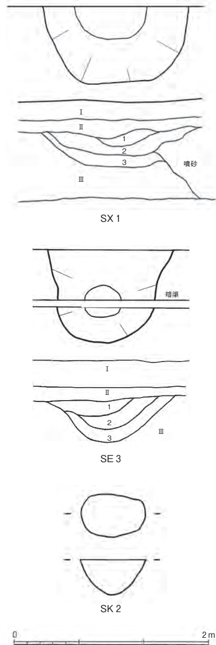
図3 遺構平面断面図(1/40)
