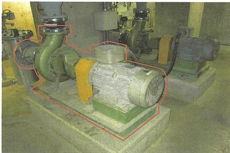
施工対象（No. 2機器冷却水循環ポンプ）
