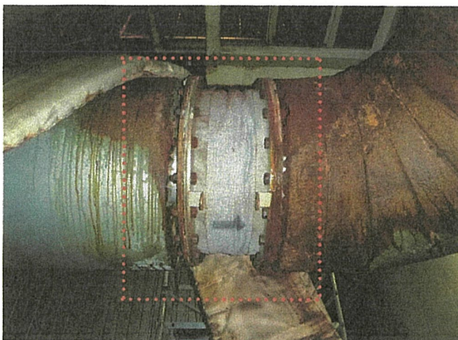
施工対象（伸縮継手及びダクト） （着手前）
