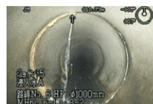
管渠のTVカメラ調査
