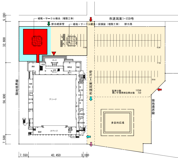
配置図 S=1:100
