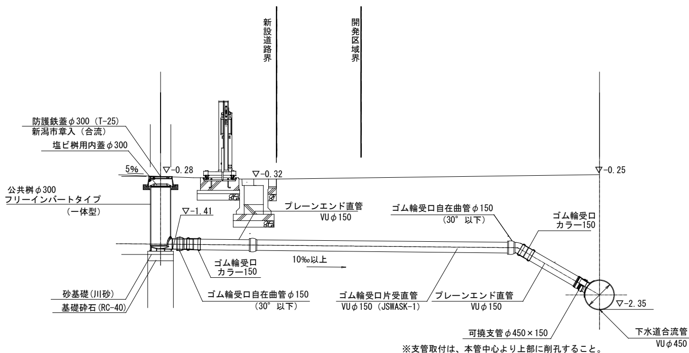
汚水取付管断面図 (北側) S=1:30
