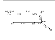
拡大図 S=1/280 (A3)
