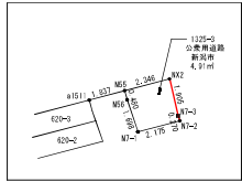
拡大図 S=1/280 (A3)
