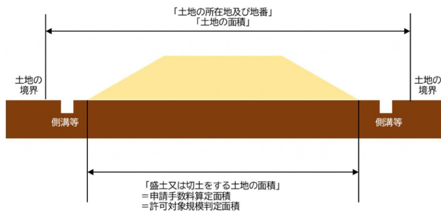
図 4-3 面積の考え方(盛土のみを行う場合)
