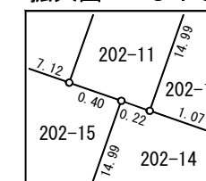
拡大図 S=1:50
