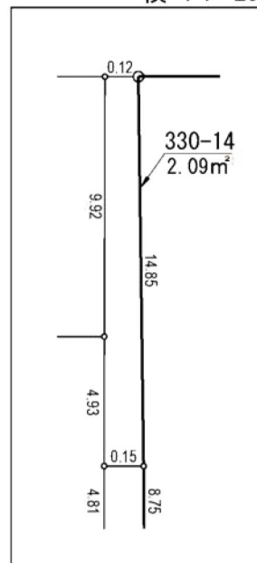
拡大図A 縦 1 : 250 横 1 : 25
