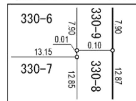
拡大図C' S=1:10
