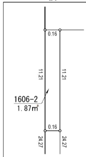
拡大図 A 縦 1 : 250 横 1 : 25
