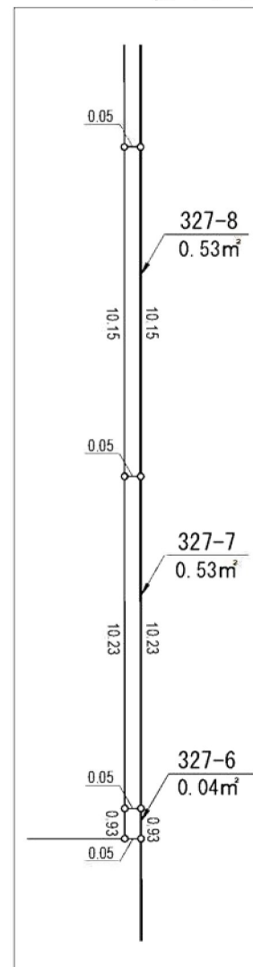
拡大図B 縦 1 : 200 横 1 : 20
