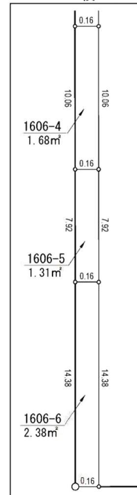
拡大図 C 縦 1 : 250 横 1 : 25
