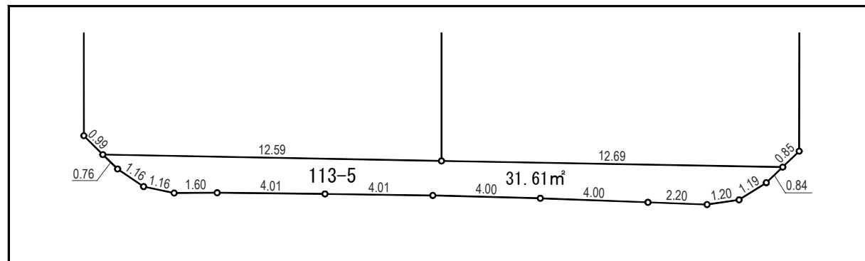
拡大図 A S=1:200
