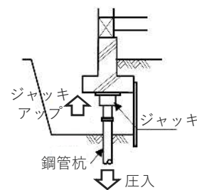
アンダーピニング工法
