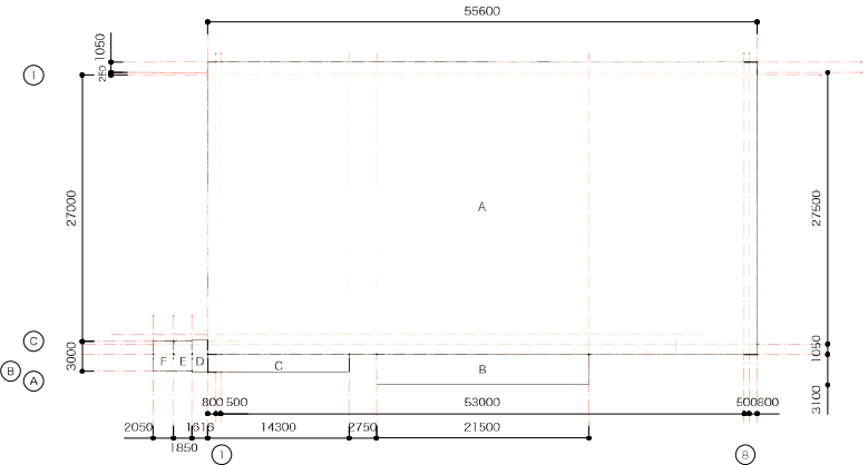
体育館建築面積求積図
