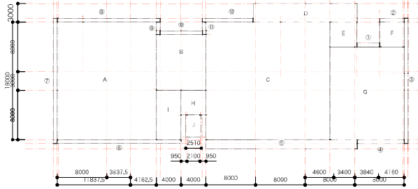
建築面積求積図
