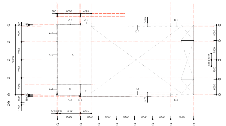
体育館2階求積図
