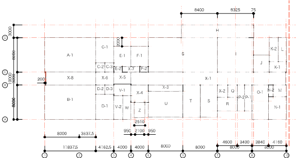
1階求積図
