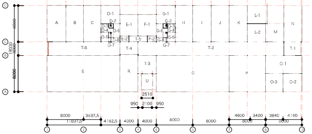
3階求積図
