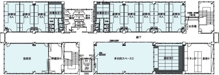
【校舎棟 4 階】
