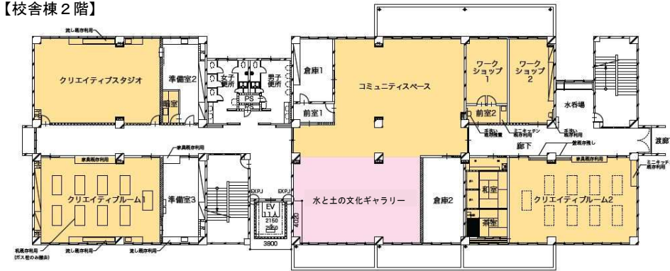
【校舎棟 2階】
