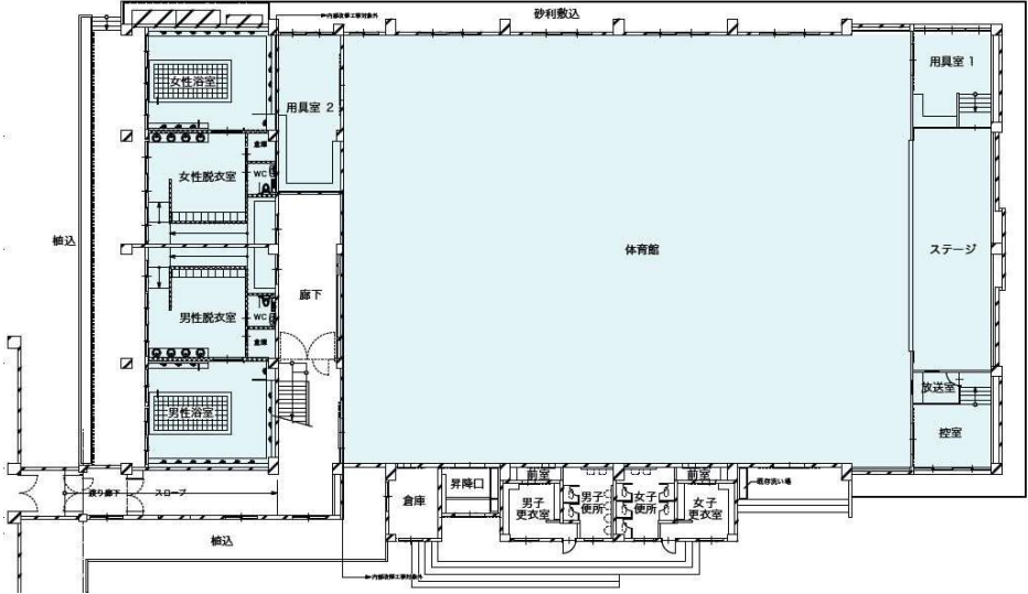
【体育館棟 1 階】
