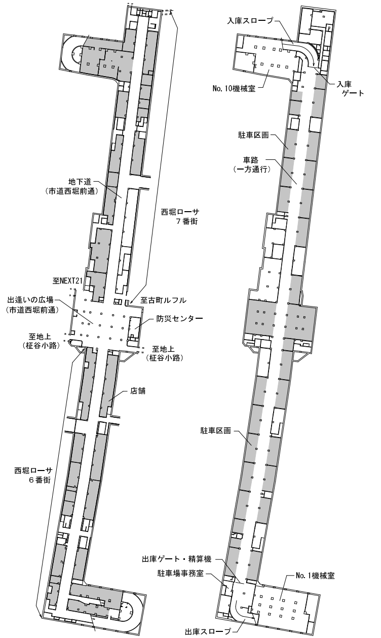
地下1階平面図 S:1/1400 (A3)
