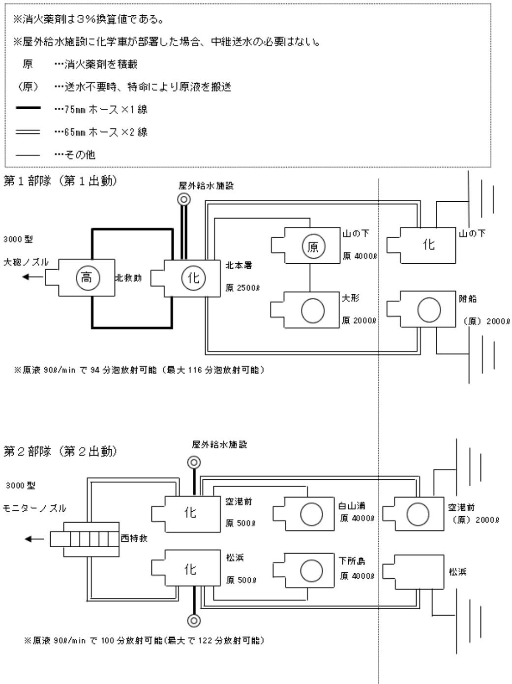
石油コンビナート等火災出動部隊編成図
