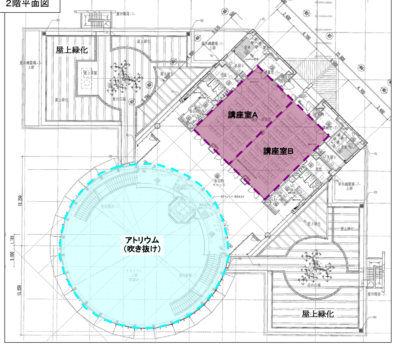
2階平面図
