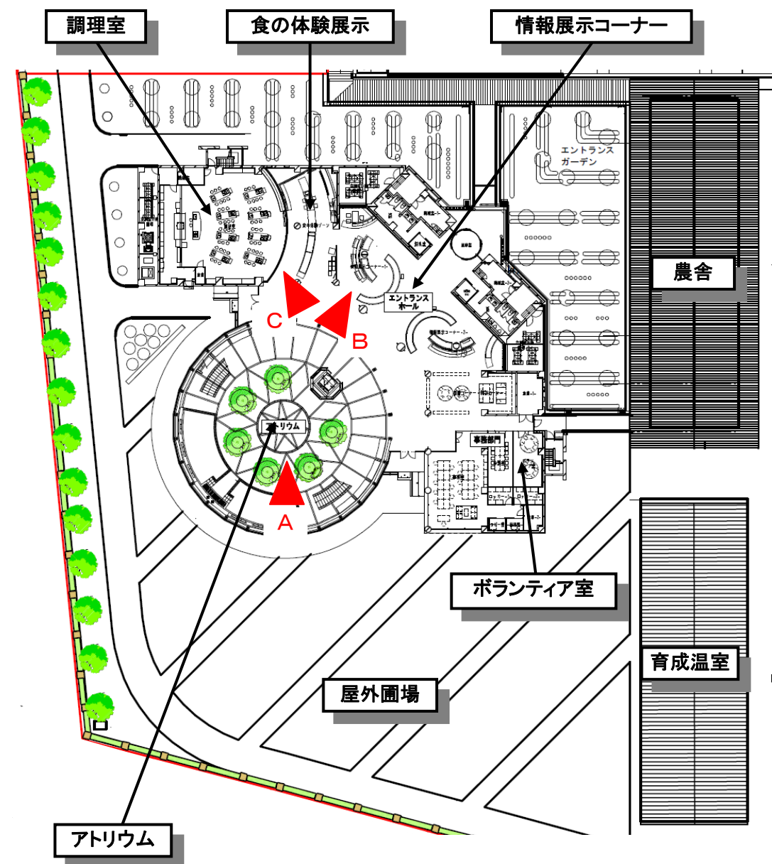
1階平面図
