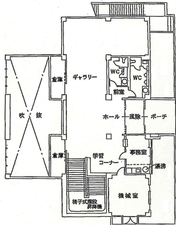
2 階平面図
