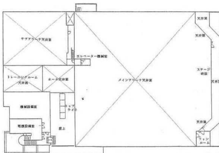
3階平面図
