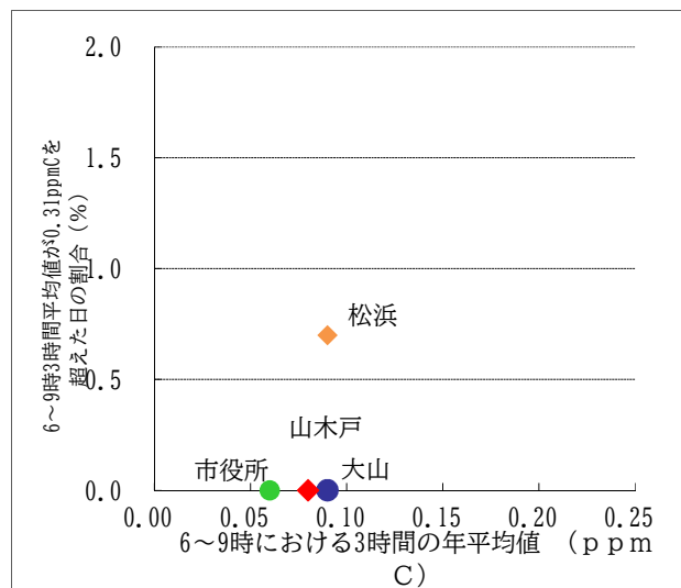
図 令和4年度における非メタン炭化水素濃度の傾向
