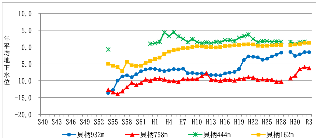
図 地下水位の経年変化(貝柄観測井)
