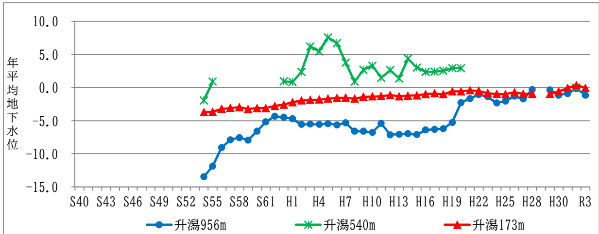
図 地下水位の経年変化(升瀉観測井)
