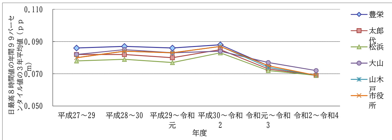
図 「日最高8時間値の年間99パーセンタイル値の3年平均値」の経年変化① (豊栄局、太郎代局、松浜局、大山局、山木戸局、亀田局)
