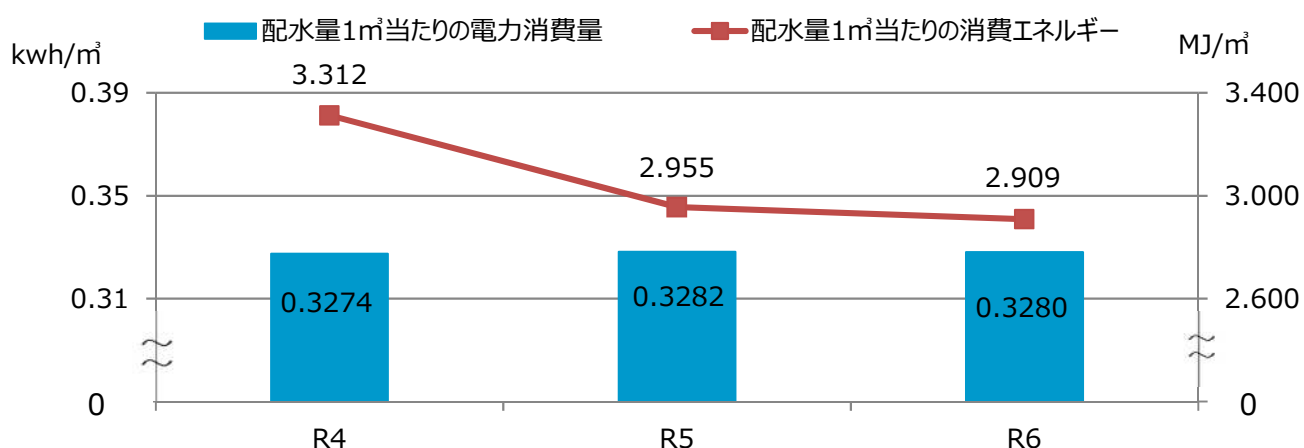
配水量1m 3 当たりの電力消費量(kwh/m 3 )・消費エネルギー(MJ/m 3 )
