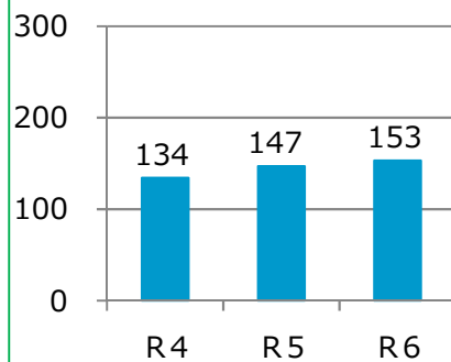
ガス使用量(千m 3 )
