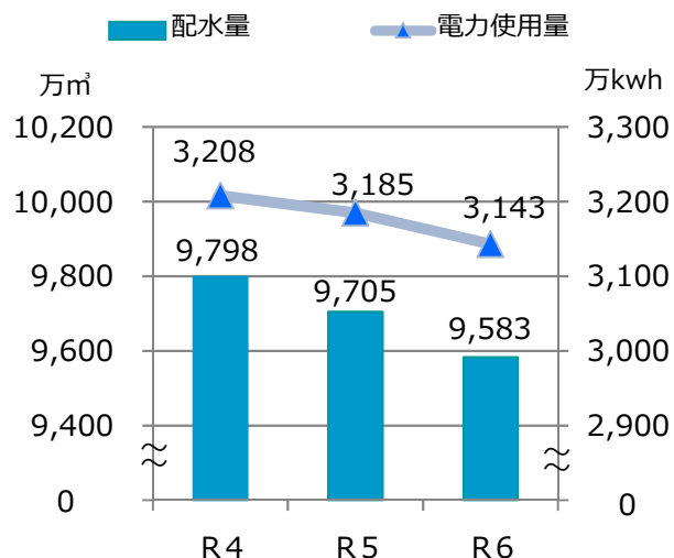
電力使用量(万kwh)と配水量(万m 3 )
