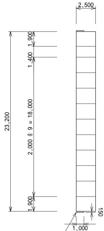
C-C'断面図
