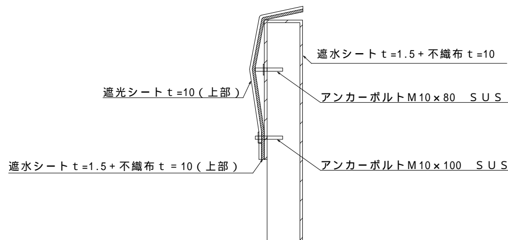
A部 シート設置詳細断面図 S=1:NON
