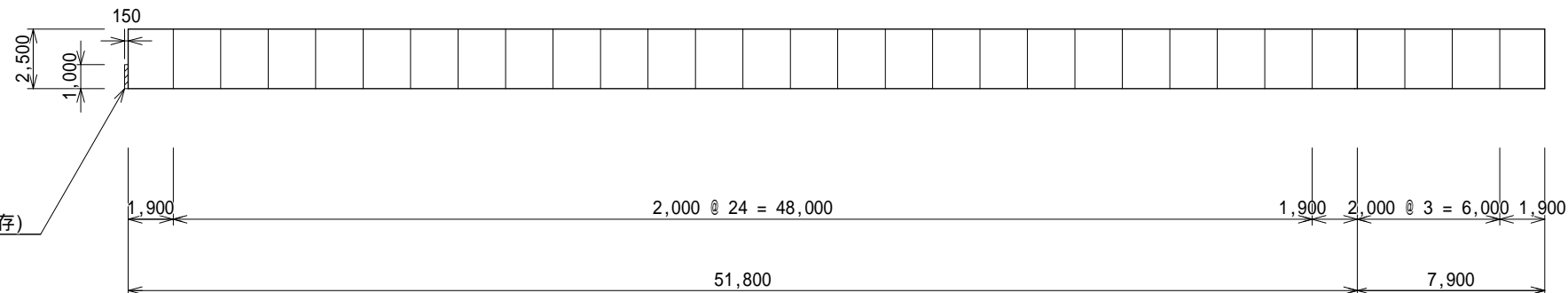
B-B'断面図
