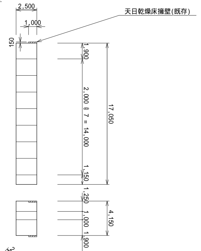
D-D'断面図
