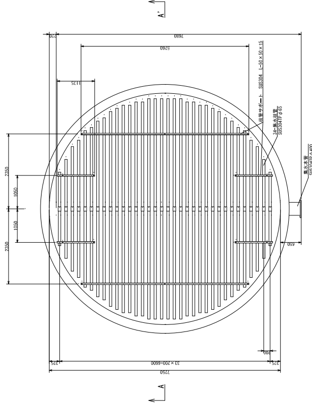
1系ろ過池1号詳細図 S=1/60
