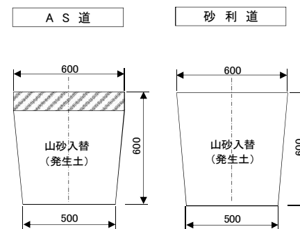
給水引き込み部・土工掘削断面 （人力掘削）
