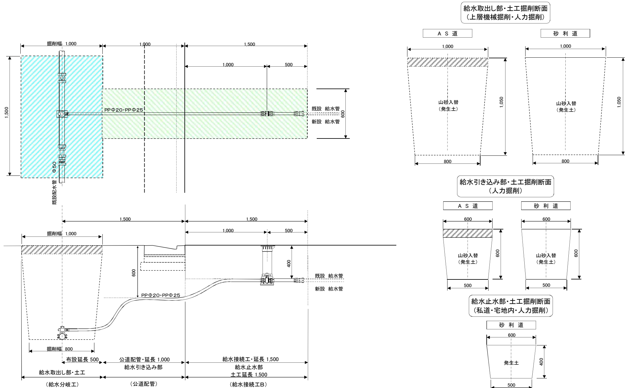
図－９ 給水接続工B（既設配水管Φ50を切り落としサドル分岐して私道・宅地内の第1止水栓付近までの給水接続に適用）
