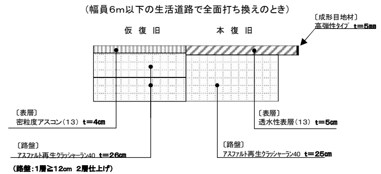
AS道 市道C断面・透水性舗装
