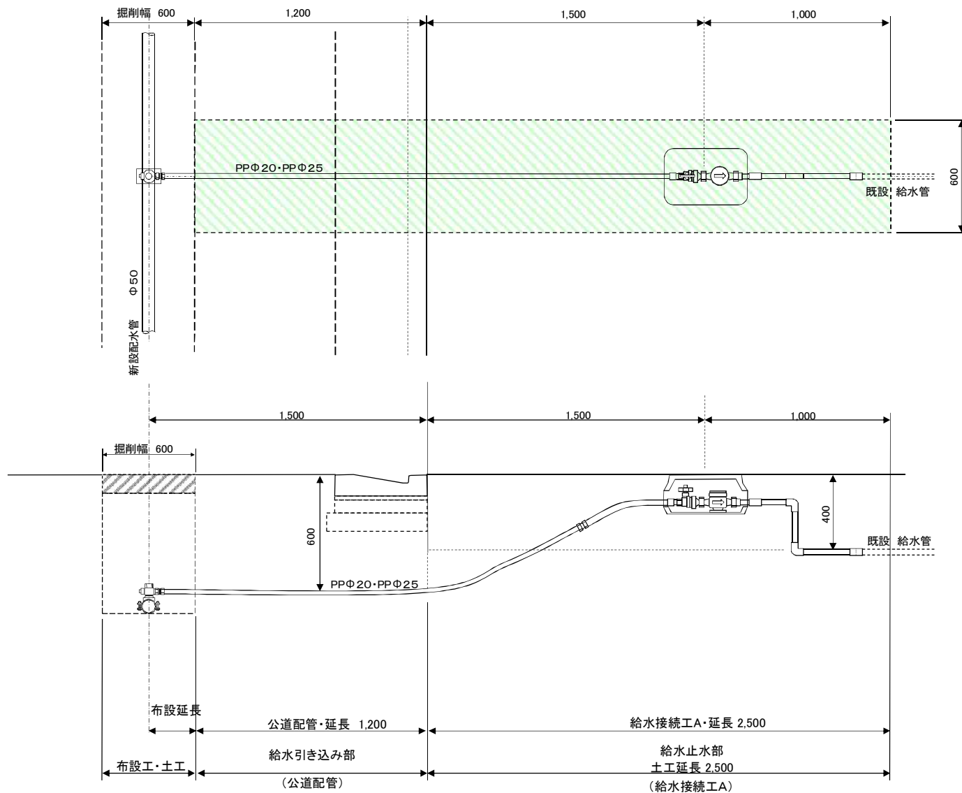
図 - 5 給水接続工A（新設配水管Φ50mmから宅地内メータまでの給水接続に適用）
