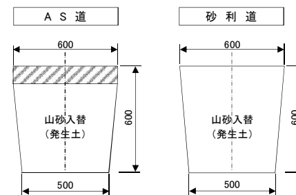
給水止水部・土工掘削断面 (宅地内・人力掘削)
