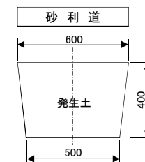
給水止水部・土工掘削断面 (宅地内・人力掘削)
