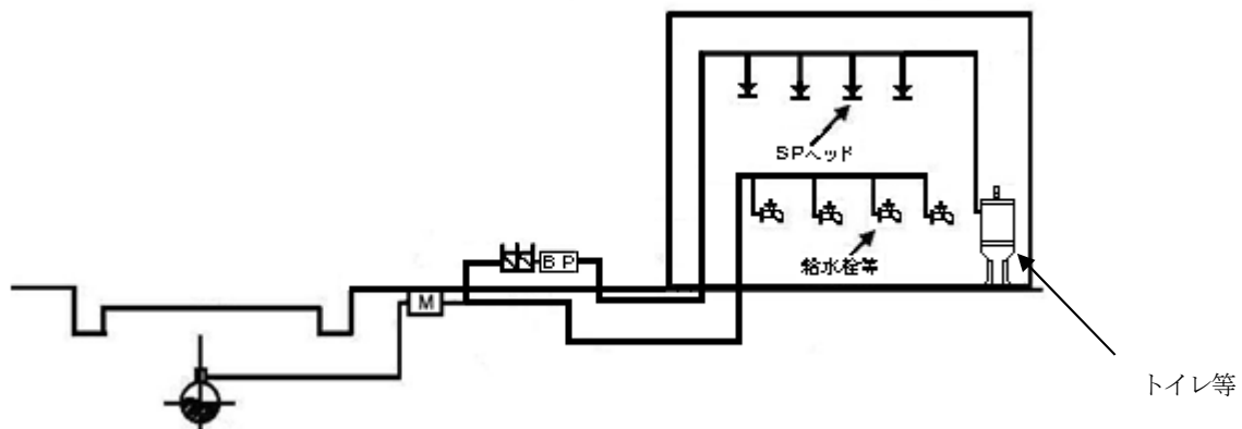
図10-3 スプリンクラーシステムのみ増圧方式
