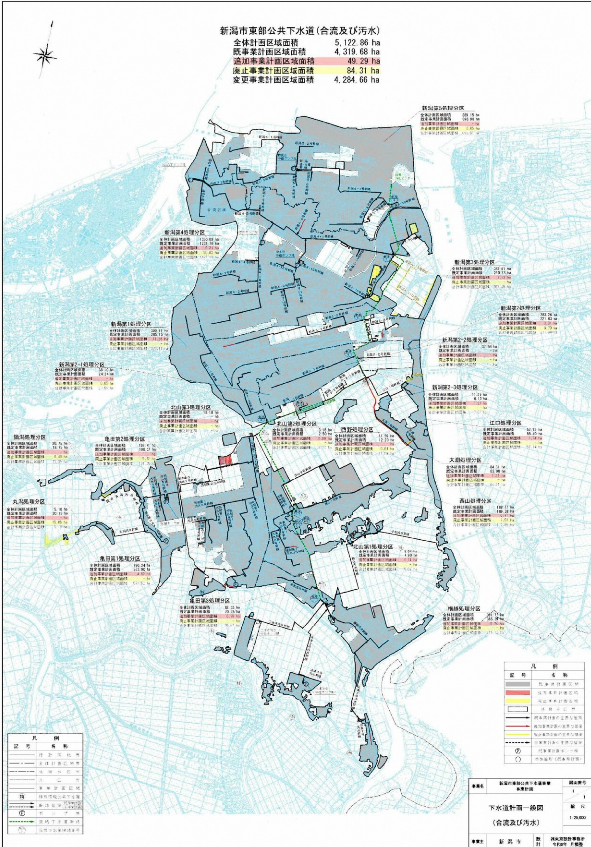
出典：令和5年度信濃川下流域下水道(新潟処理区)関連新潟市東部公共下水道事業全体計画 図表 3.1-5 東部処理区の下水道計画一般図(合流及び分流汚水)
