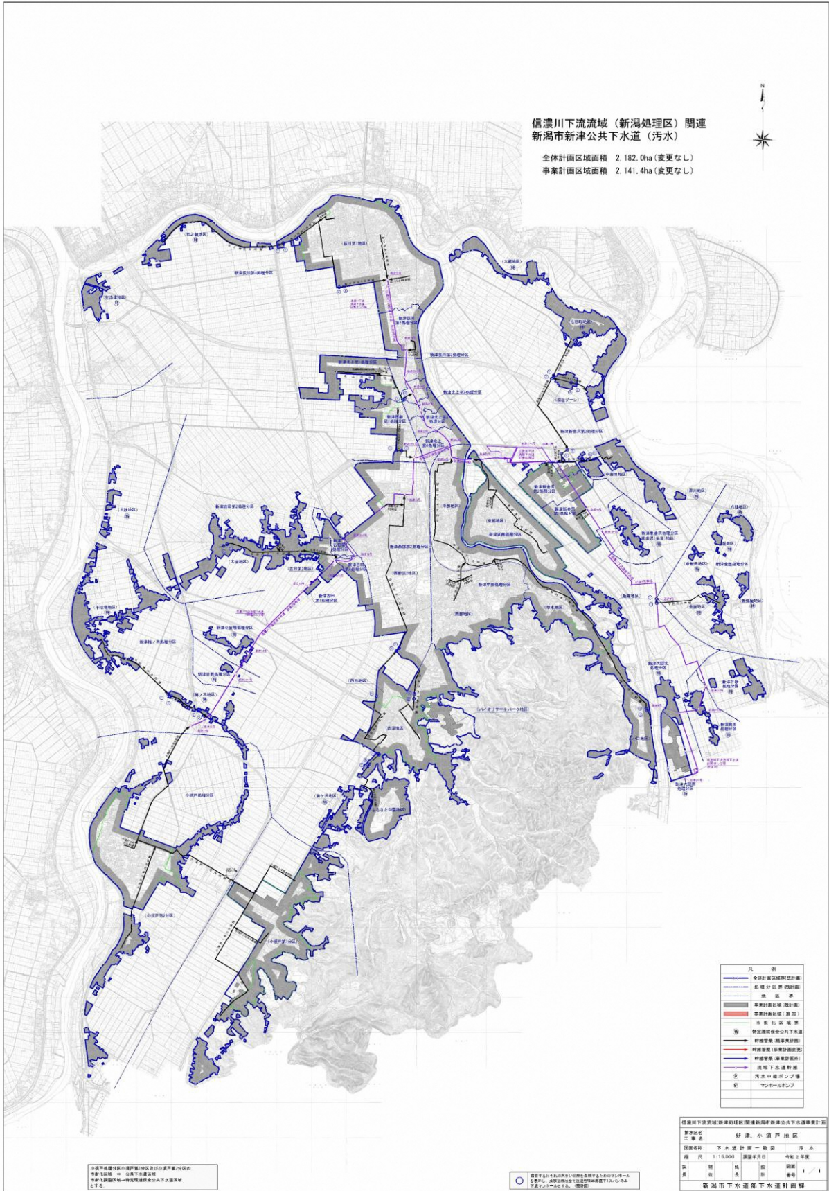
出典：令和3年度信濃川下流域下水道(新潟処理区)関連新潟市新津公共下水道事業計画 変更協議書 図表 3.1-7 新潟処理区の下水道計画一般図(污水)
