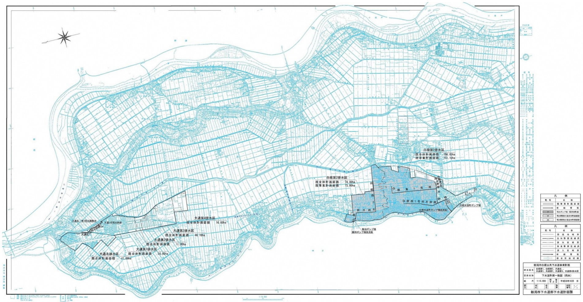
出典：平成30年度新潟市白根公共下水道（白根処理区）変更事業計画書 図表 3.1-4 白根処理区の下水道計画一般図（雨水）
