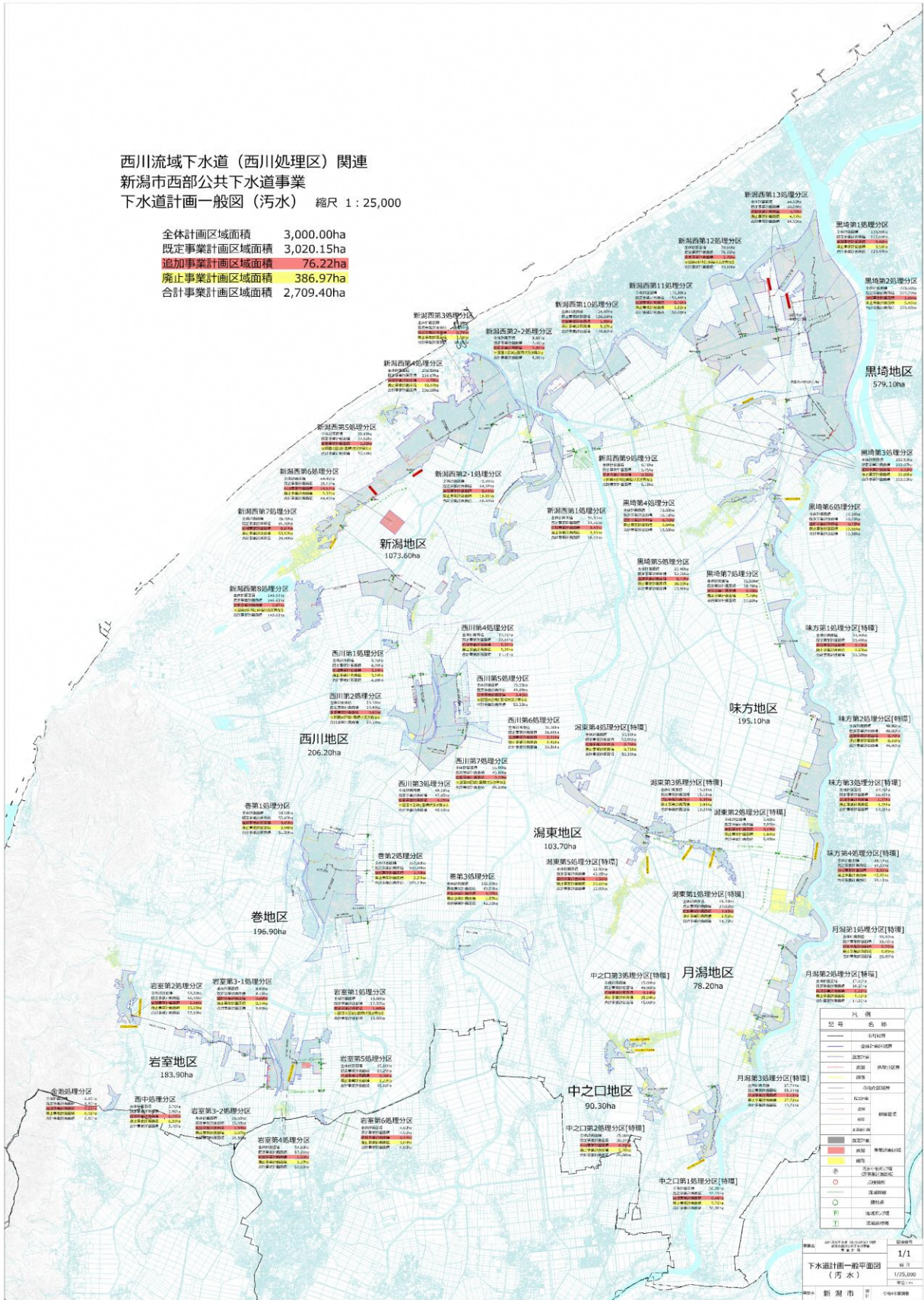
出典：令和4年度西川流域下水道（西川処理区）関連新潟市西部公共下水道事業事業計画 図表 3.1-13 西部処理区の下水道計画一般図（污水）
