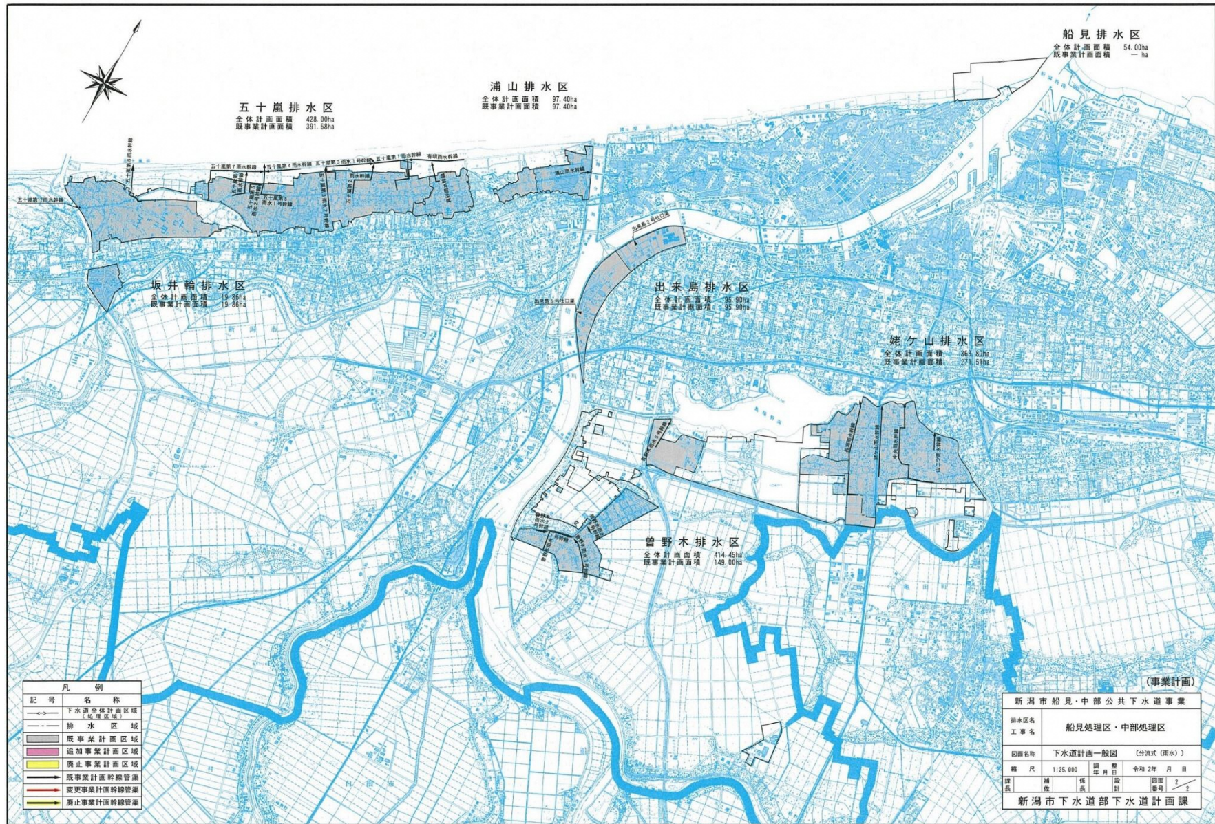
図表 2.2-4 船見・中部処理区の下水道計画一般図（雨水）
