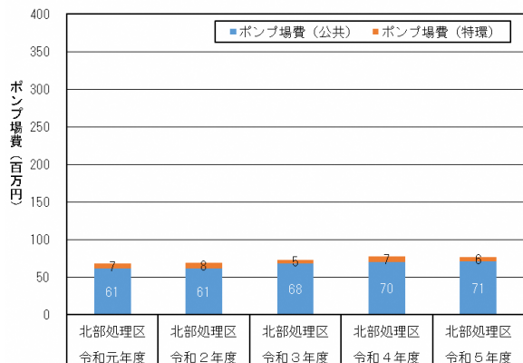
(e) 北部処理区
