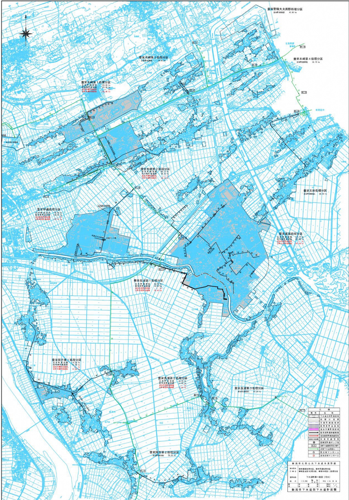
出典：令和3年度 阿賀野川流域下水道（新井郷川処理区）関連新潟市北部公共下水道 事業計画変更協議申請書 図表 3.1-11 北部処理区下水道計画一般図（雨水、豊栄地区）
