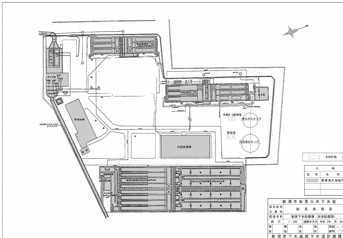
図表 2.2-1 施設配置図（船見下水処理場）
