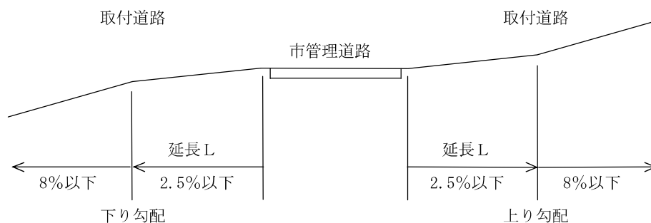
（参考図）取付道路の縦断勾配
