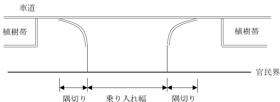
（参考図）乗り入れ口 平面図
