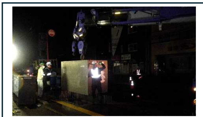
地中構造物（電力地上機器ます）設置状況（夜間工事）
