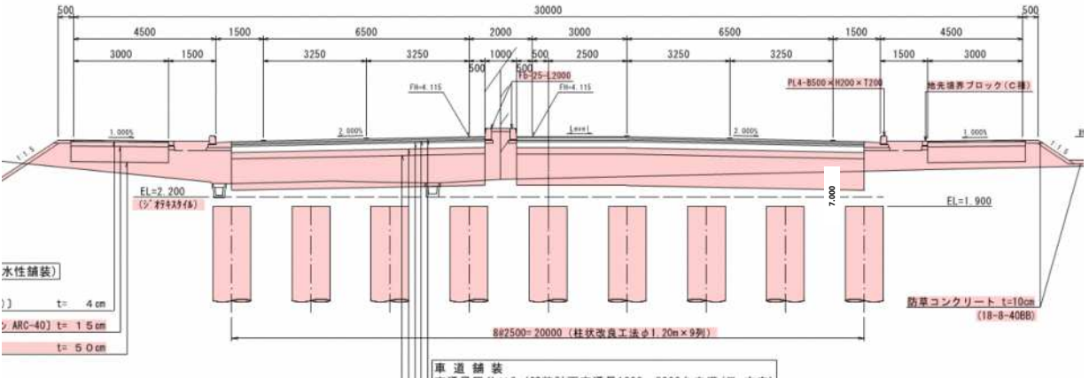
【 標 準 断 面 図 】
