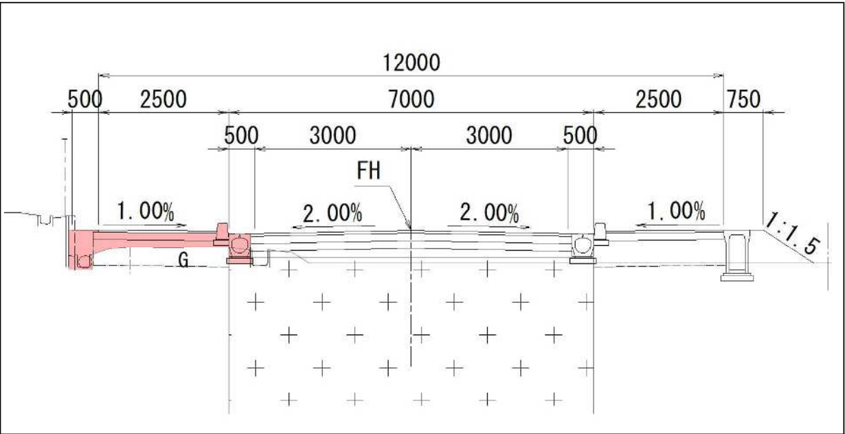
標準横断面図
