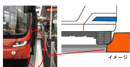
写真 38 バリアレス縁石の設置 (バス停のバリアフリー化)
