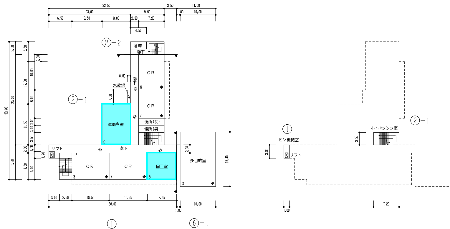
屋階平面図
