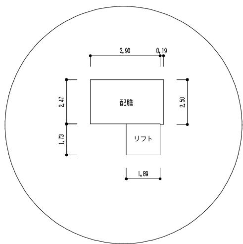
2階平面図
