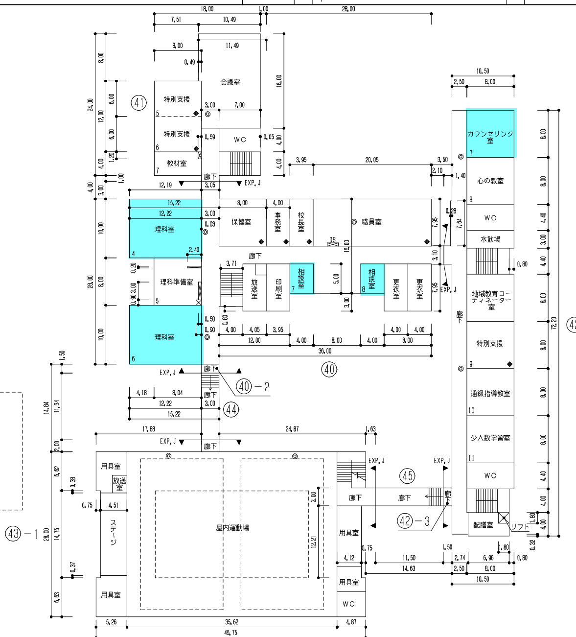
2 階 平 面 図
