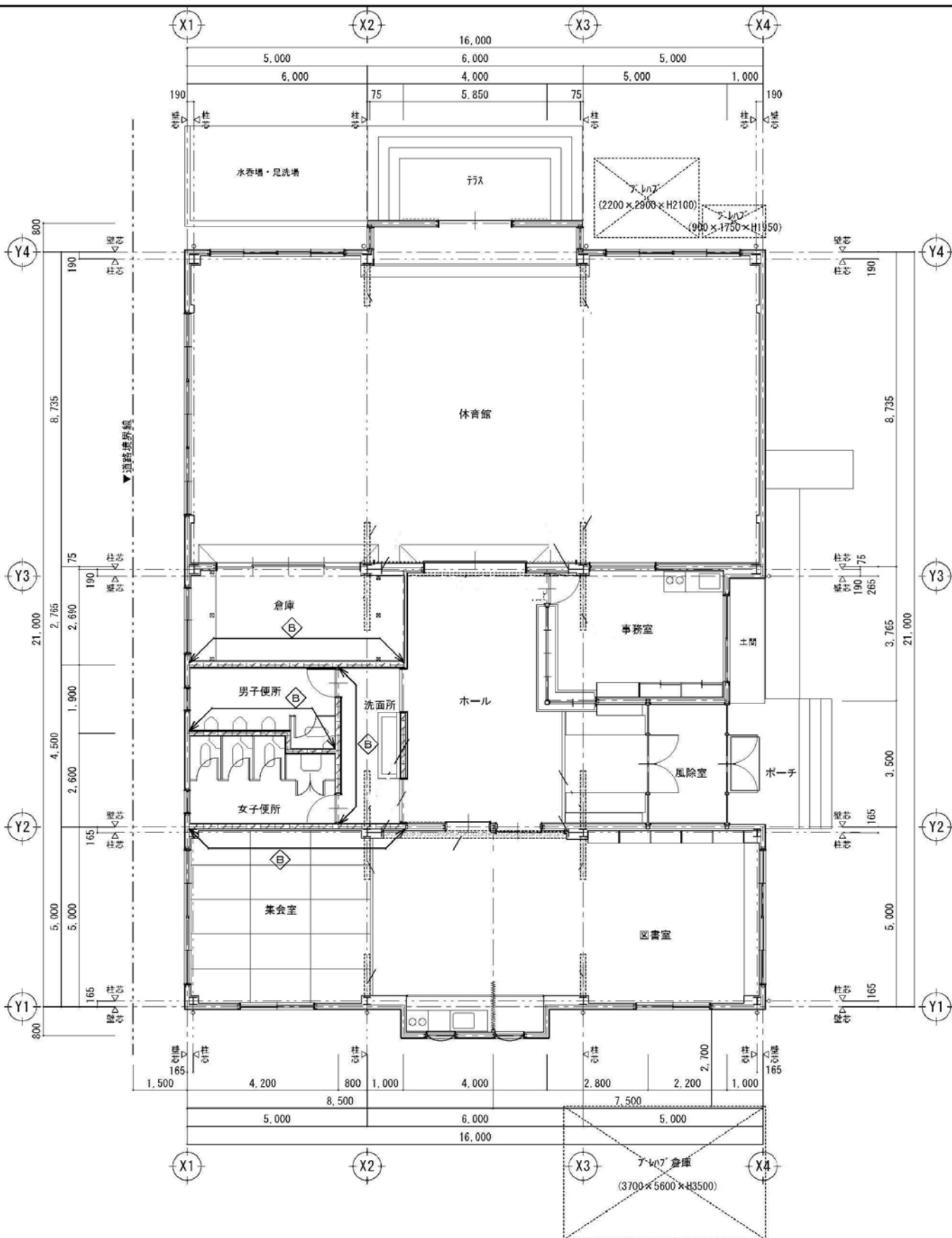
1階平面図 (改修後) S=1:100
