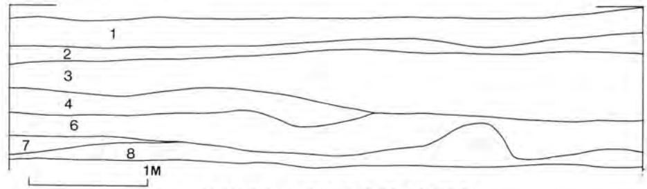
第4図の2 No.8トレンチ西側土層断面図
