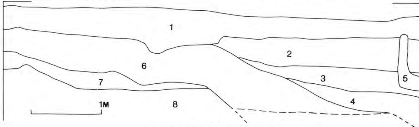
第4図の4 No.57トレンチ北側土層断面図
