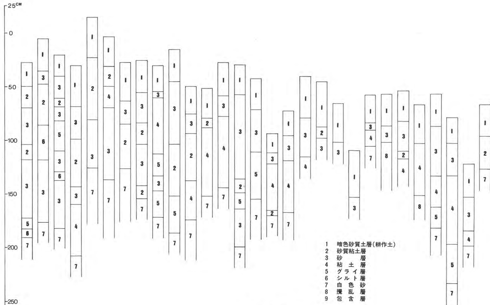
第5図 土層柱状図
