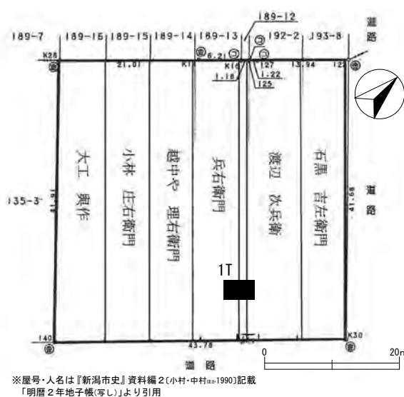
図6 第27次調査トレンチ位置図 (1/800)
