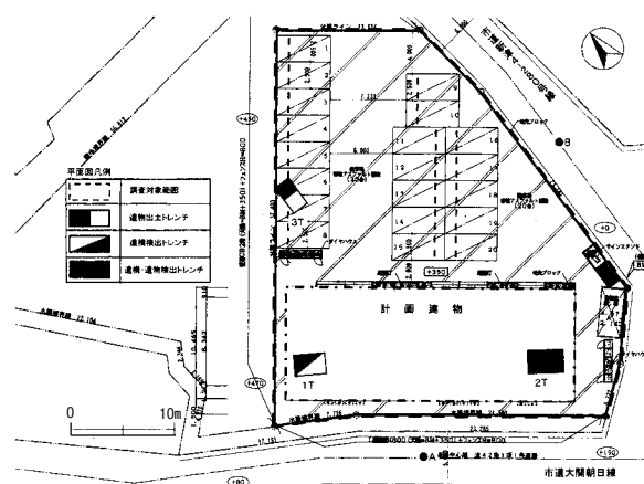
図2 トレンチ位置図 (1/800)
