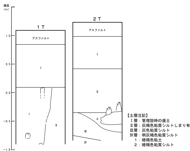
図4 第23次調査土層柱状図 (1/40)
