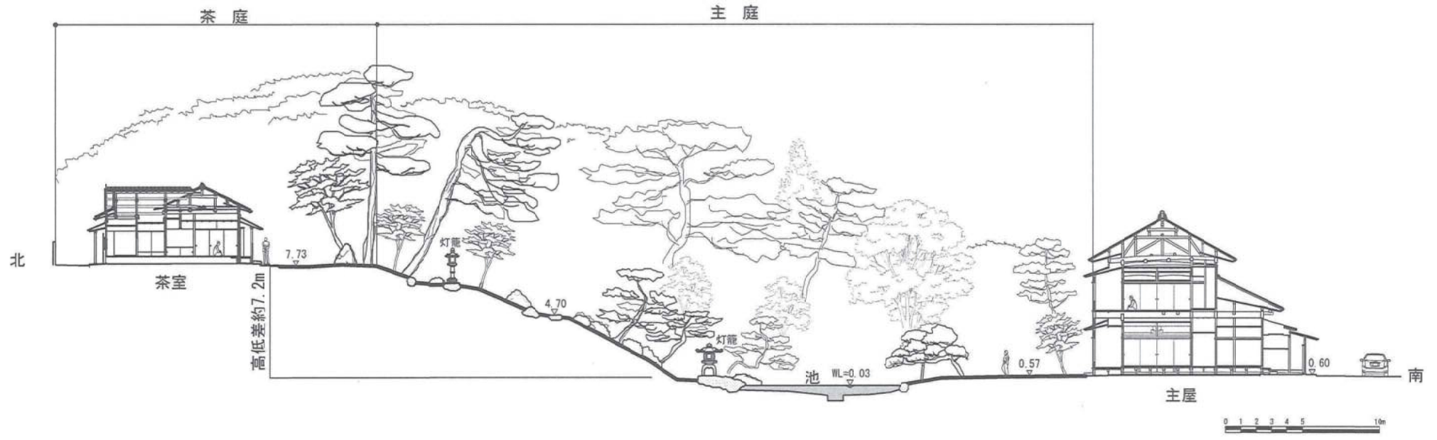
主要部断面図
