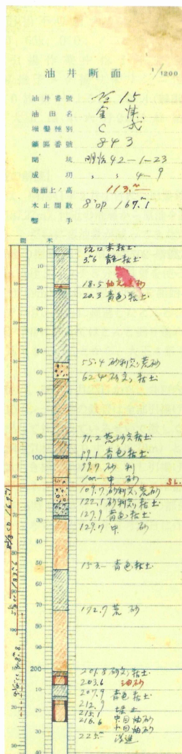
油井断面図 C15号井 (左: 表上部 右: 表下部) (中野家文書/市撮影)
