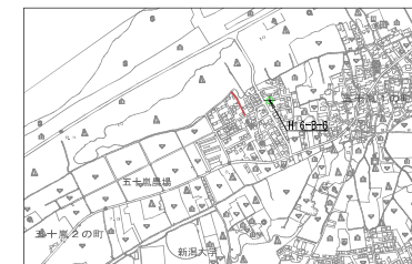
位置図 S=1:10,000
