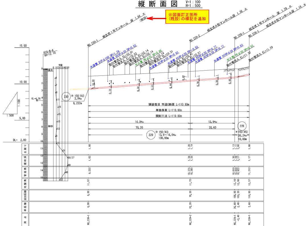
縦断面図 V=1:100 H=1:500
