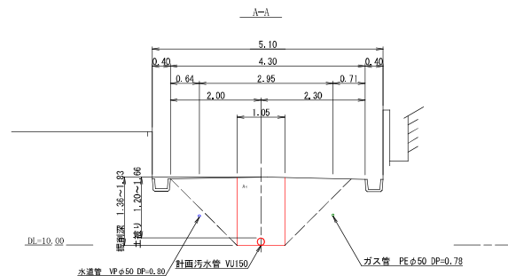
標準横断面図 S=1:50
