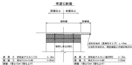
舗装復旧断面図 S=1:20
