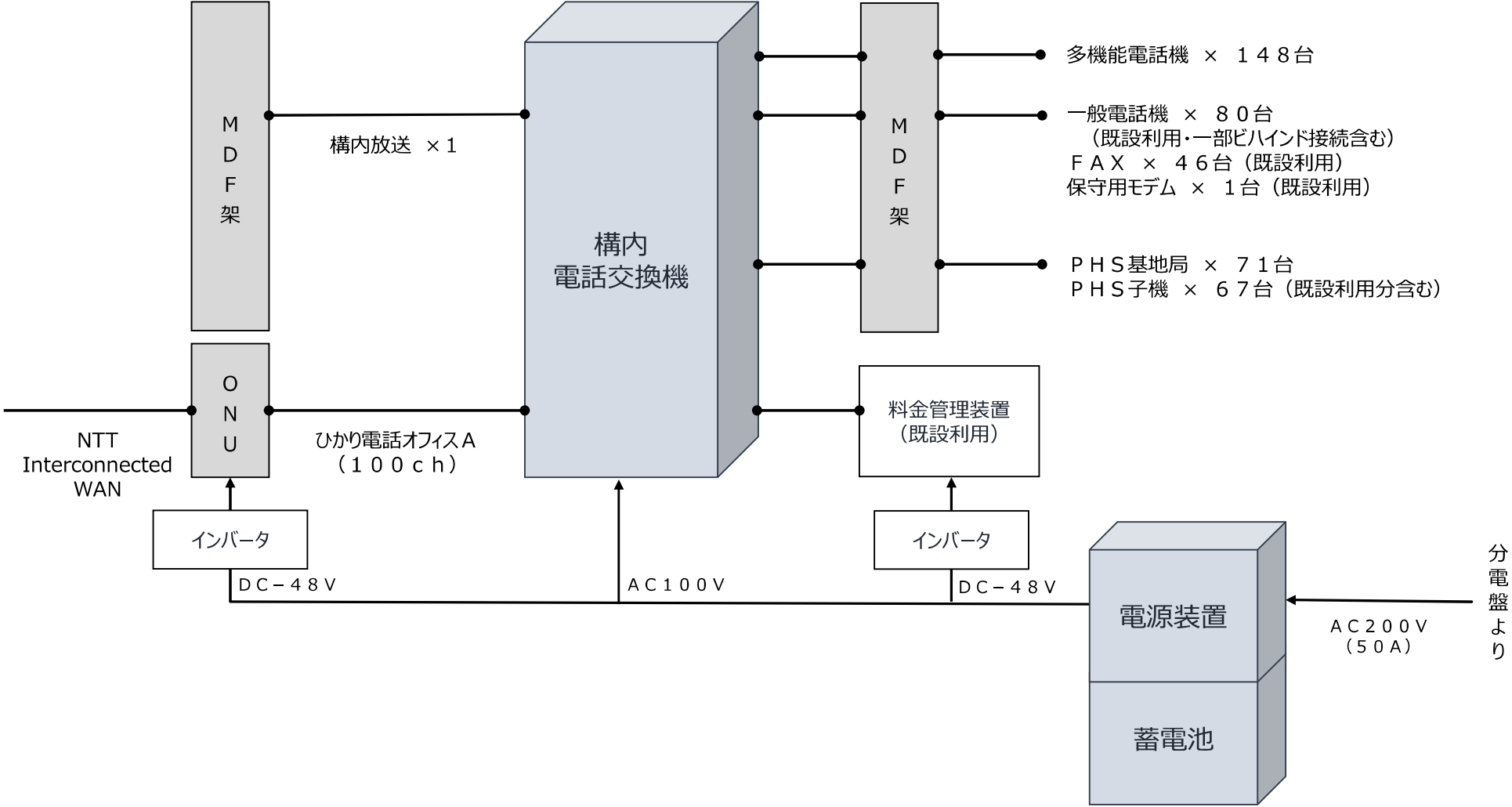
【別図 1】システム構成図（中継方式図）
