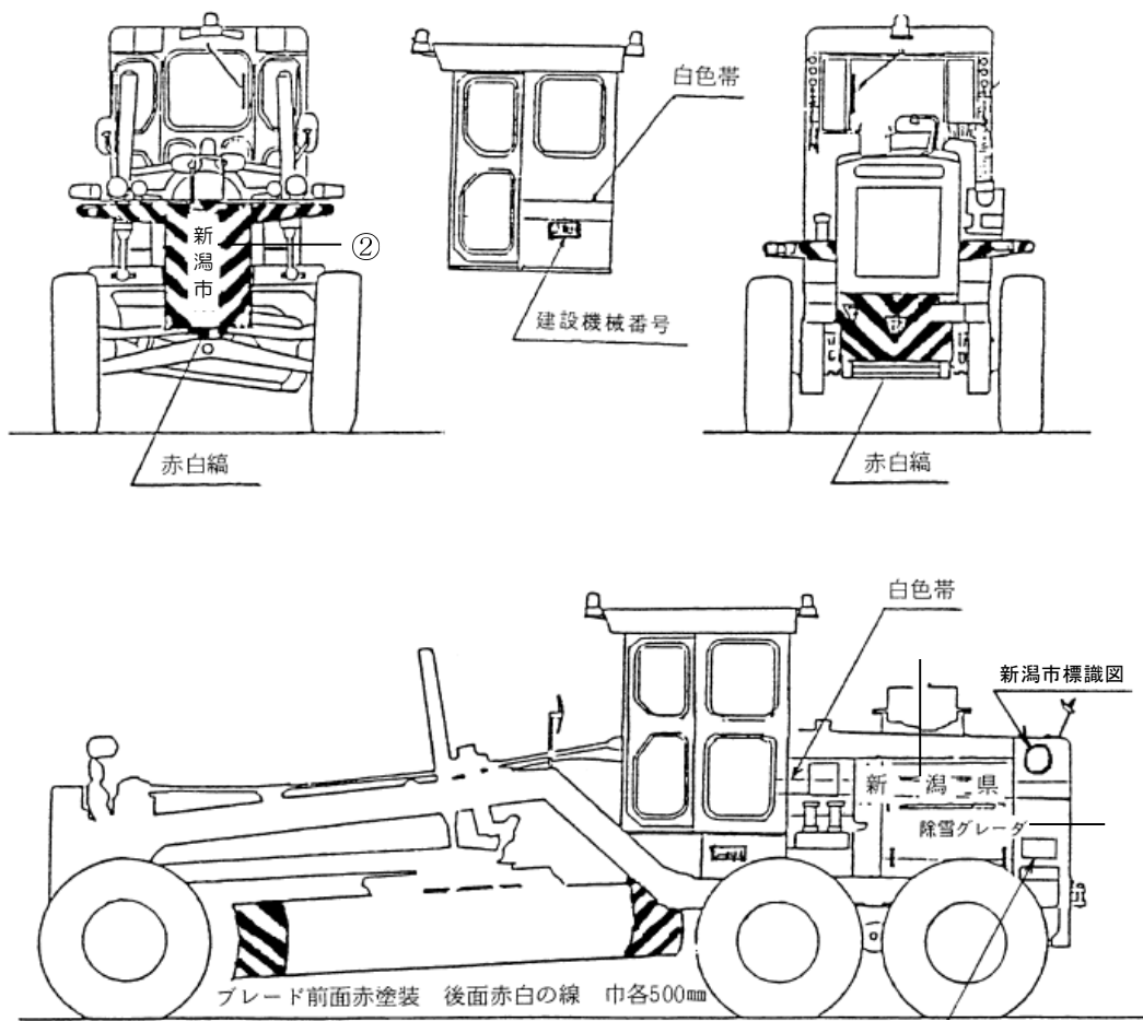
図 1 - 除雪機械表示箇所図
