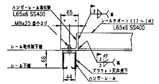
ハンガーレール取付詳細
